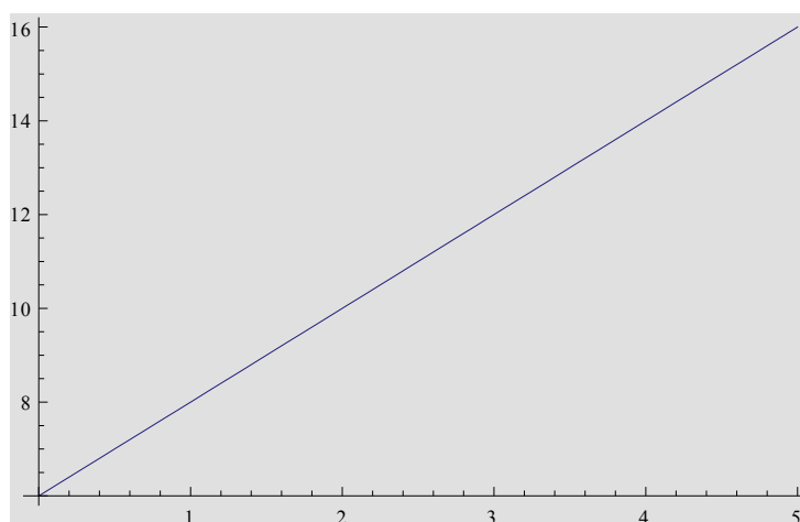
Фигура 5. Графично представяне на закона за скоростта v = 6 + 2t
