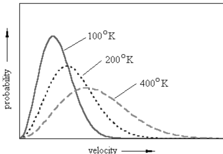
Фигура 1. Разпределение на молекулите на един газ по скорости: Закон на Максвел, който за течности не е валиден
