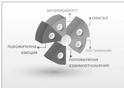
Фигура 2. Модел на теория за благополучието ПЕРМА, адаптирана по M. Seligman (2017)
