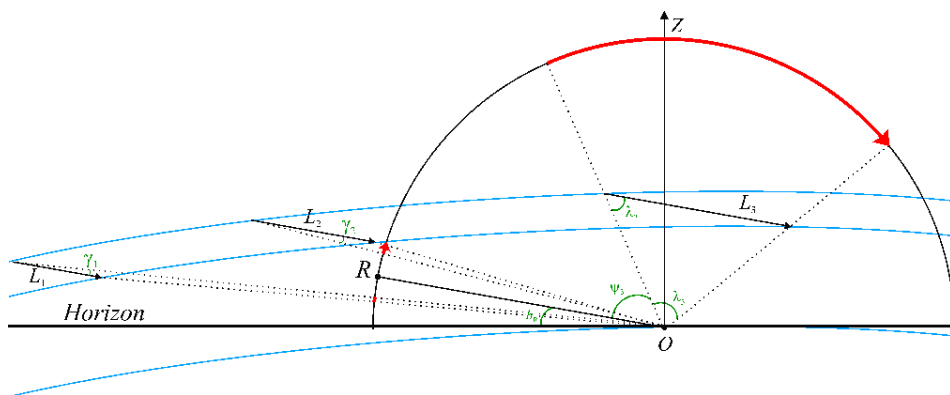
Фигура 10. Когато радиантът се намира близо до хоризонта, ефектът с проекции на дължини и скорости се подсилва поради различната отдалеченост на метеора до наблюдателя
