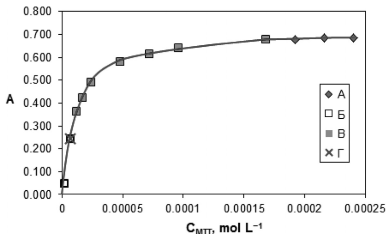
Фиг.5. Крива на насищане с 3-(4,5-диметил-2-тиазол)-2,5-дифенил-2Н-тетразолиев бромид (МТТ) в системата Ga(III) – 4-(2-пиридилазо)-резорцинол – МТТ – вода – хлороформ (Stojnova & Gavazov, 2012). C_{Ga(III)} = 7,2 \times 10^{-6} \text{ mol L}^{-1} , C_{PAR} = 1,6 \times 10^{-4} \text{ mol L}^{-1} , pH=6.5 , \lambda=515 \text{ nm} , l=1
