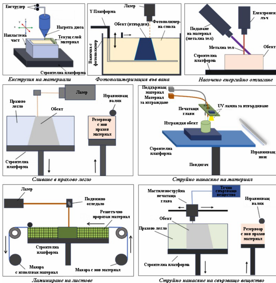
Фигура 2. Принципи на 7-те вида адитивни процеси (Ukwaththa et al., 2024)
